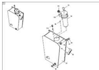
ЕТВ-0000010132, Масло
