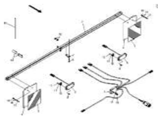
ETB-022561, Освещение для движения по дорогам Condor 12001-C/15001-C (1)
