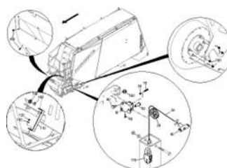
ЕТВ-0000004195, Бункер 7800L / навесные детали (2)
