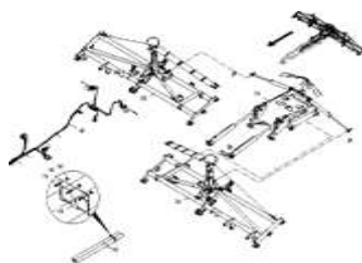
ЕТВ-0000004106, Задний модуль Condor 12001
