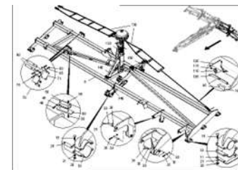
ЕТВ-022557, Боковая рама слева Condor 15001
