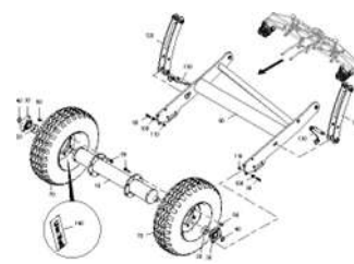
ETB-022564, Комплект копирующее колесо
