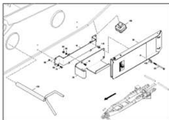
ЕТВ-0000004034, Базовая машина Condor 12001-C, 15001-C противооткатные упоры
