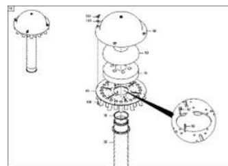
ЕТВ-0000009648, Распределительная головка без технологической колеей, 24 выхода
