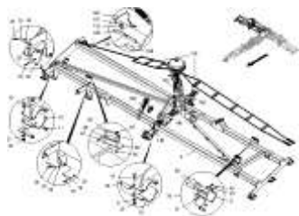
ЕТВ-022556, Боковая рама справа Condor 15001
