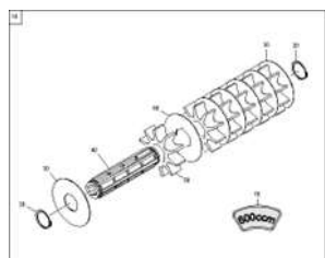
ЕТВ-0000007840, Дозирующий ролик 600 куб.см
