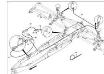
ЕТВ-0000004997, Кабельный комплект Digitroll распределительная головка 2
