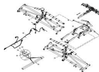
ЕТВ-022555, Задний модуль Condor 15001
