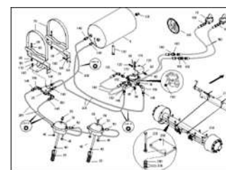
ЕТВ-0000004817, Ось с двухконтурной пневматической тормозной системой (40 км/ч)
