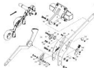
ЕТВ-0000004903, Кронштейн сошника в сборе
