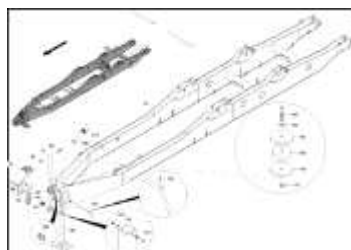
ЕТВ-0000004120, Базовая машина Condor 15001-С, основная рама
