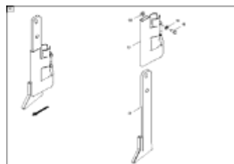
ЕТВ-0000009669, Плоские зубья
