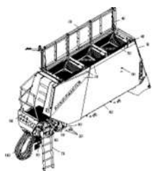
ЕТВ-0000009561, Бак 7800Л
