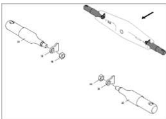
ЕТВ-0000009718, Палец нижней тяги Кат. K700 для самостоятельной сборки
