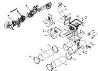
ЕТВ-0000010938, Конвейерная линия Condor механическая (2)
