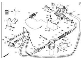
ЕТВ-0000007653, Набор приспособлений для жидких удобрений Condor (1)
