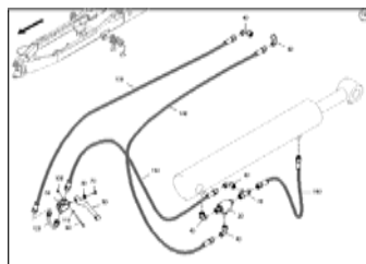
ЕТВ-0000006692, Гидравлические детали колесного молота трактора
