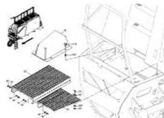
ЕТВ-0000004190, Бункер 7800L / сетчатая решетка, решетчатая подножка, защитная решетка
