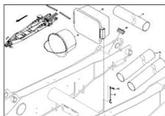
ЕТВ-0000004035, Базовая машина Condor 12001-С, 15001-С навесные детали
