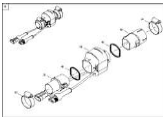
ЕТВ-0000008898, Датчик контроля посевной линии Slue
