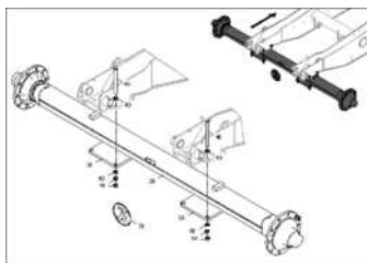
ЕТВ-0000009721, Ось без тормозов, для контролируемого земледелия
