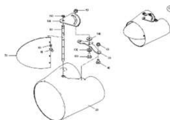
ЕТВ-0000009516, Воздухораспределитель 200-125-125
