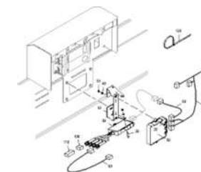
ЕТВ-0000006177, Контроль высева Digitroll базовый пакет
