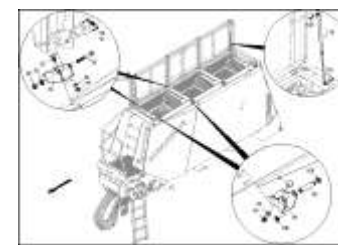
ЕТВ-0000004077, Бункер 7800Л / напорная крышка накладки
