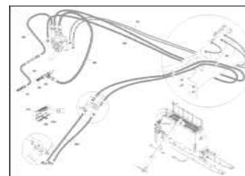
ETB-0000004464, Загрузочный шнек Citan Condor / MBG гидравлика шланги
