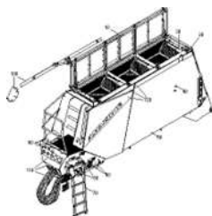
ЕТВ-0000010881, Бак 7800 л
