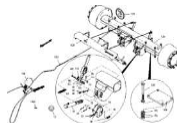
ЕТВ-022488, Мост с гидравлической тормозной системой 12001-C/15001-C 8000L (1)
