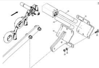
ЕТВ-0000001013, Опора
