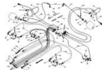
ЕТВ-022576, Гидр. детали задний модуль Condor 15001
