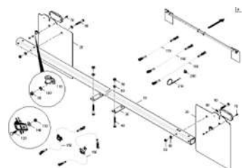
ETB-0000004349, Освещение CN 1 (2)
