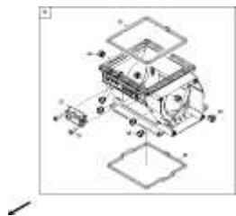
ЕТВ-0000010231, Корпус с одним дозатором справа
