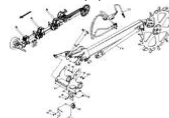
ЕТВ-0000010967, Конвейерная линия Condor механическая, привод на хвостовое колесо
