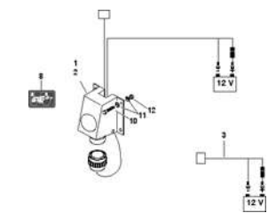
ETB-022584, Основное оборудование ISOBUS
