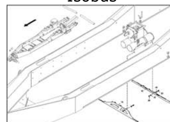
ЕТВ-0000004039, Базовая машина Condor 12001-С, 15001-С направляющая ванны
