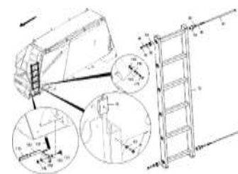
ЕТВ-0000004094, Бункер 7800Л / лестница
