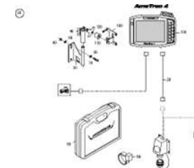
ETB-0000008868, Операторский терминал ISOBUS AmaTron 4
