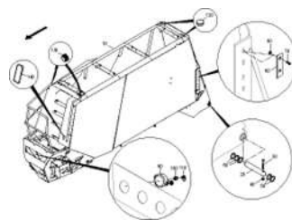
ЕТВ-0000004192, Бункер 7800L / напорный бункер
