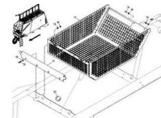
ЕТВ-0000004189, Бункер 7800L / сетчатый ящик
