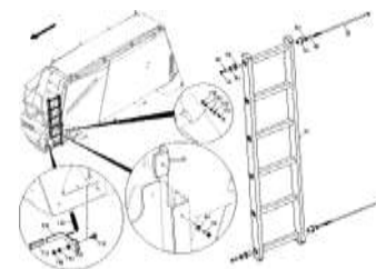
ЕТВ-0000004193, Бункер 7800L / лестница
