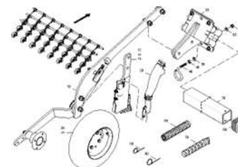
ЕТВ-0000001015, Набор сошников 48 313
