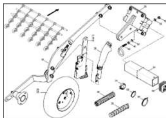
ЕТВ-0000000997, Набор сошников 36 333
