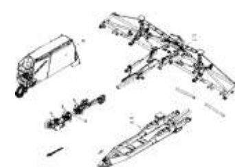
ЕТВ-0000004030, Базовая машина Condor 12001-C / 15001-C
