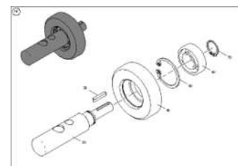
ЕТВ-0000009058, Механический привод с 02.2021
