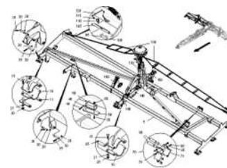
ЕТВ-022556, Боковая рама справа Condor 15001
