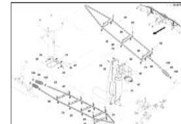
ЕТВ-022546, Монтажные детали распределительная головка 7500 слева
