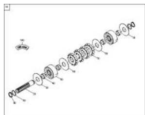
ЕТВ-0000007807, Дозирующий ролик 100 см 3
