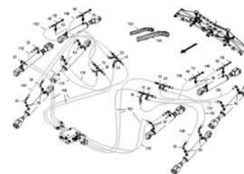
ЕТВ-0000004175, Гидравлические детали Condor 12001 консоль
