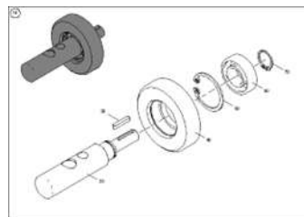
ETB-0000009057, Механический привод до 02.2021
