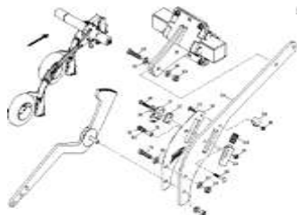
ЕТВ-0000000593, Кронштейн сошника в сборе
