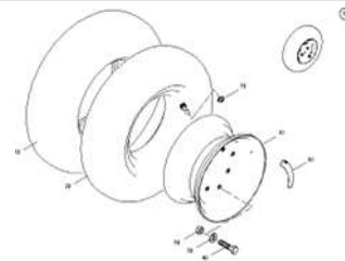
ЕТВ-0000001005, Выбег колесо с пневматической шиной
