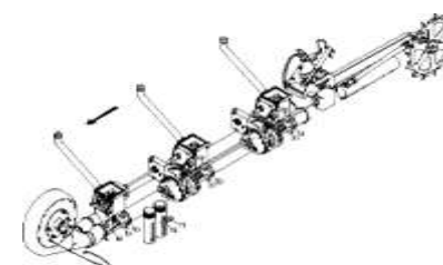
ЕТВ-0000010971, Конвейерная линия Condor механическая, фольгирование
