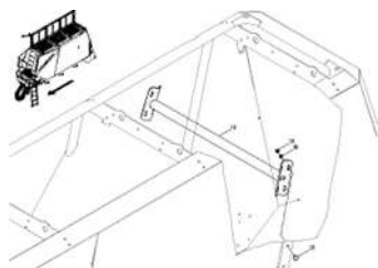
ЕТВ-0000004191, Бункер 7800L / распорка
