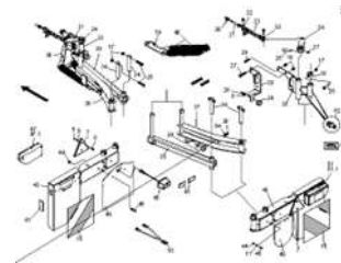
ETB-022562, Освещение для движения по дорогам Condor 12001-C/15001-C (2)
