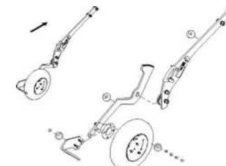
ЕТВ-0000009502, Базовый сошник ConTeC Pro с колесной держателем Solo
