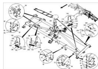
ЕТВ-0000004114, Боковая рама слева Condor 12001
