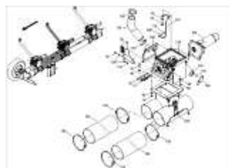
ЕТВ-0000010920, Конвейерная линия Condor электрическая (2)
