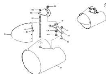
ЕТВ-0000009516, Воздухораспределитель 200-125-125
