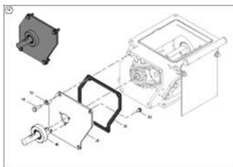
ETB-0000009056, Подкомплект механического привода до 02.2021
