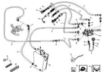
ЕТВ-022580, Привод вентилятора от бортовой гидросистемы
