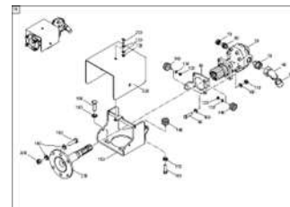
ЕТВ-022578, Гидр. детали насадной насос K700 35CCM
