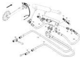
ЕТВ-0000001536, Колесо с почвозацепами гидравлические детали
