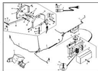
ЕТВ-0000004475, Пакет электроники Citan Condor датчик рабочего положения / Isobus
