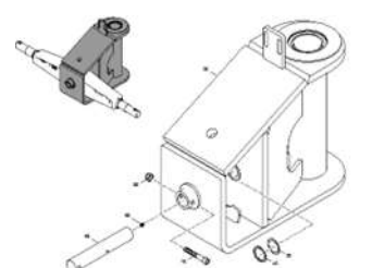
ЕТВ-0000004048, Condor 12001-C, 15001-C дышло
