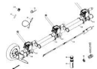
ETB-0000010925, Конвейерная линия Condor, электрическая
