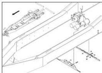
ЕТВ-0000004039, Базовая машина Condor 12001-C, 15001-C направляющая ванны
