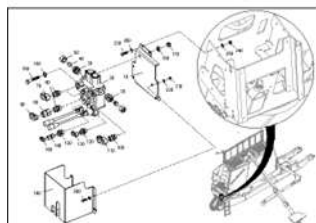
ETB-0000004458, Заправочный винт Citan Condor / MBG панель управления гидравликой
