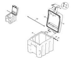
ЕТВ-0000004115, Бокс для хранения в сборе
