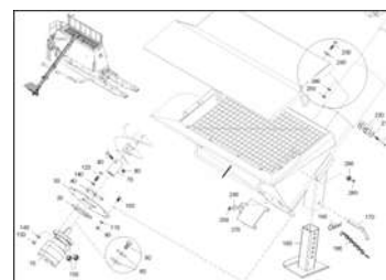
ETB-0000004453, Загрузочный шнек Citan Condor / MBG загрузочный шнек (2)
