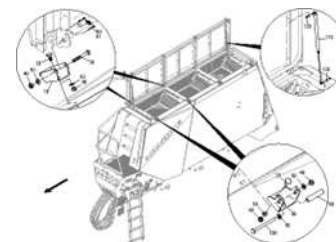
ЕТВ-0000004188, Бункер 7800L / напорная крышка накладки
