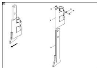
ЕТВ-0000009667, Крутые зубья
