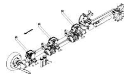
ETB-0000010971, Конвейерная линия Condor механическая, фольгирование
