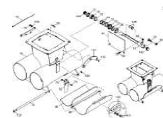
ЕТВ-0000000988, Двойной шлюз 125
