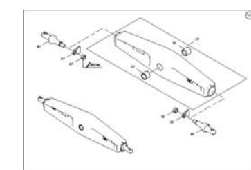
ЕТВ-0000007633, Поперечная балка поезда Cat 3
