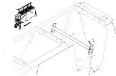
ЕТВ-0000004086, Бункер 7800Л / распорка
