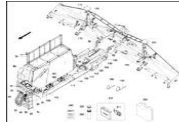
ЕТВ-0000004841, Базовая машина Condor 12001-C / 15001-C наклейки, принадлежности
