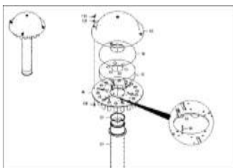
ЕТВ-0000009643, Распределительная головка без технологической колеей, 18 выходов
