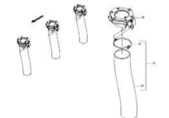
ЕТВ-0000004234, Быстрое опорожнение напорного бункера
