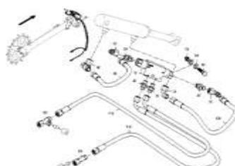
ЕТВ-0000006639, Секция конвейера 12001-15001-C / привод хвостового колеса
