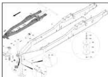
ЕТВ-0000004041, Базовая машина Condor 12001-С, основная рама
