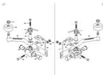
ЕТВ-0000004146, Переключающие клапаны складывание слева и справа
