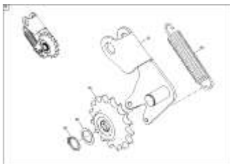
ЕТВ-0000010977, Регулятор цепи
