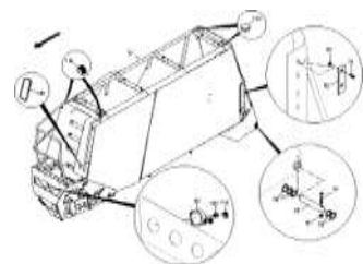
ЕТВ-0000004192, Бункер 7800L / напорный бункер
