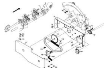
ЕТВ-0000005006, Приводные валы / подающая линия Condor мех.
