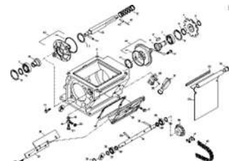
ЕТВ-022550, Однократное дозирование 2.0 Привод вправо
