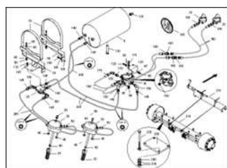
ЕТВ-0000004816, Ось с двухконтурной пневматической тормозной системой
