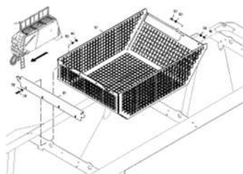
ЕТВ-0000004081, Бункер 7800Л / сетчатый ящик
