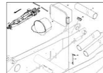
ЕТВ-0000004035, Базовая машина Condor 12001-C, 15001-C навесные детали
