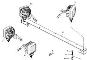
ETB-022560, Светодиодное рабочее освещение 4 элем.
