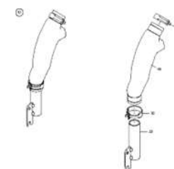
ЕТВ-0000001011, Воздухоотделитель
