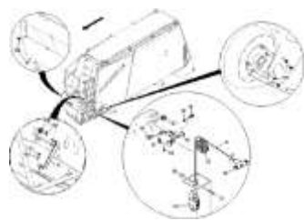
ЕТВ-0000004195, Бункер 7800L / навесные детали (2)
