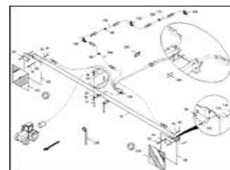
ETB-0000007983, Освещение Condor / Citan 01 (1)
